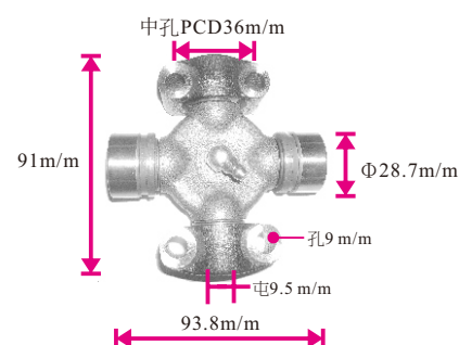
37201-26600-71 TOYOTA 8FD25 GUKO-8F
