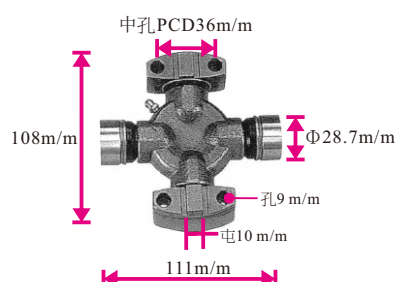
37201-23000/23320-71 TCM FD25 T3 TOYOTA 5/6/7FD25 KOMATSU 鏟土機 GUKO - 4C (GUT - 26)
