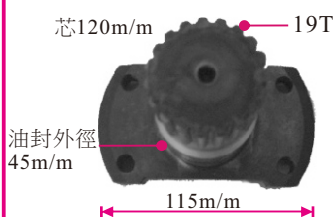
差速器
