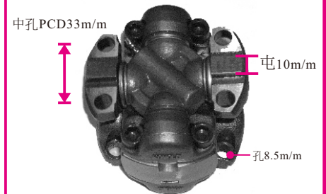
TCM SHOVELLER (鏟土機) (四孔無牙) GUKO-3
