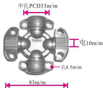
DAEWOO FD25 TCM 725/743 BOB CAT 33.34x79m/m G5-2117X(GUKO-1) 四邊孔無牙 (GUKO-2)
