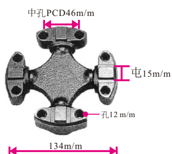
24023-30301 TCM FD35 GUTC - 2
