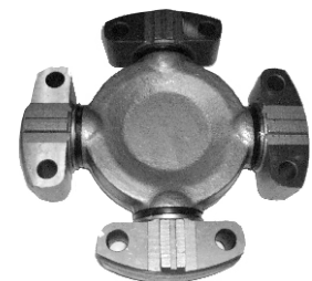
KOMATAU 鏟土機 71.44x209.62m/m C5-9016X
