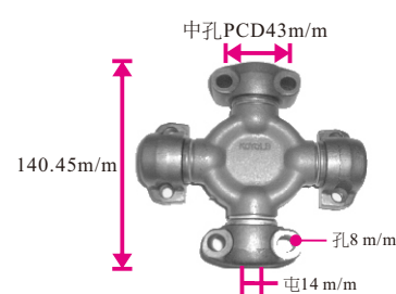
25073-30299 TCM FD35 GUTC - 1
