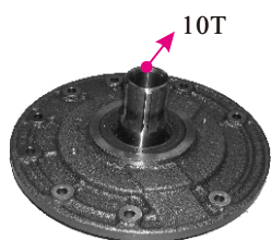
32630-23330-71 TOYOTA 7FD25 邦浦齒輪 UJ-5011
