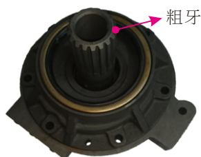
91324-07401A MITSUBISHI S4E 走路邦浦 UJ-5077
