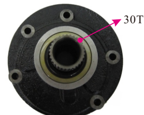
12N53-80321 TCM C3/T3 3T (C240) 30齒(5孔螺絲) 外徑154mm UJ-5058
